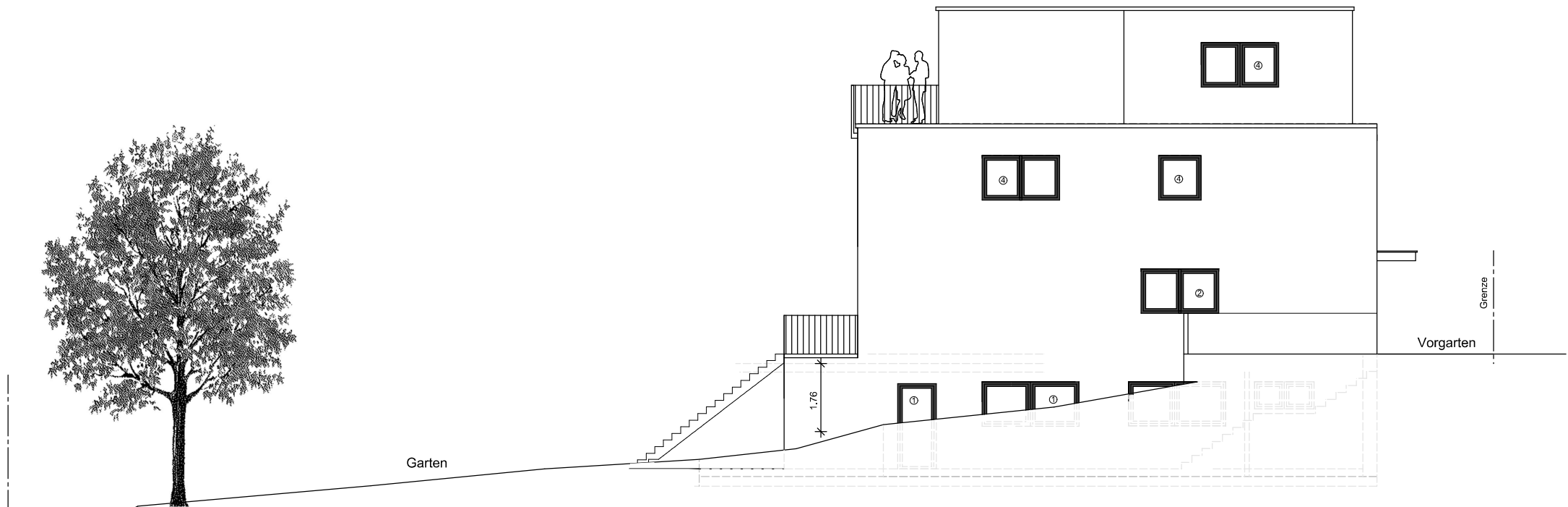
Ansicht Osten
