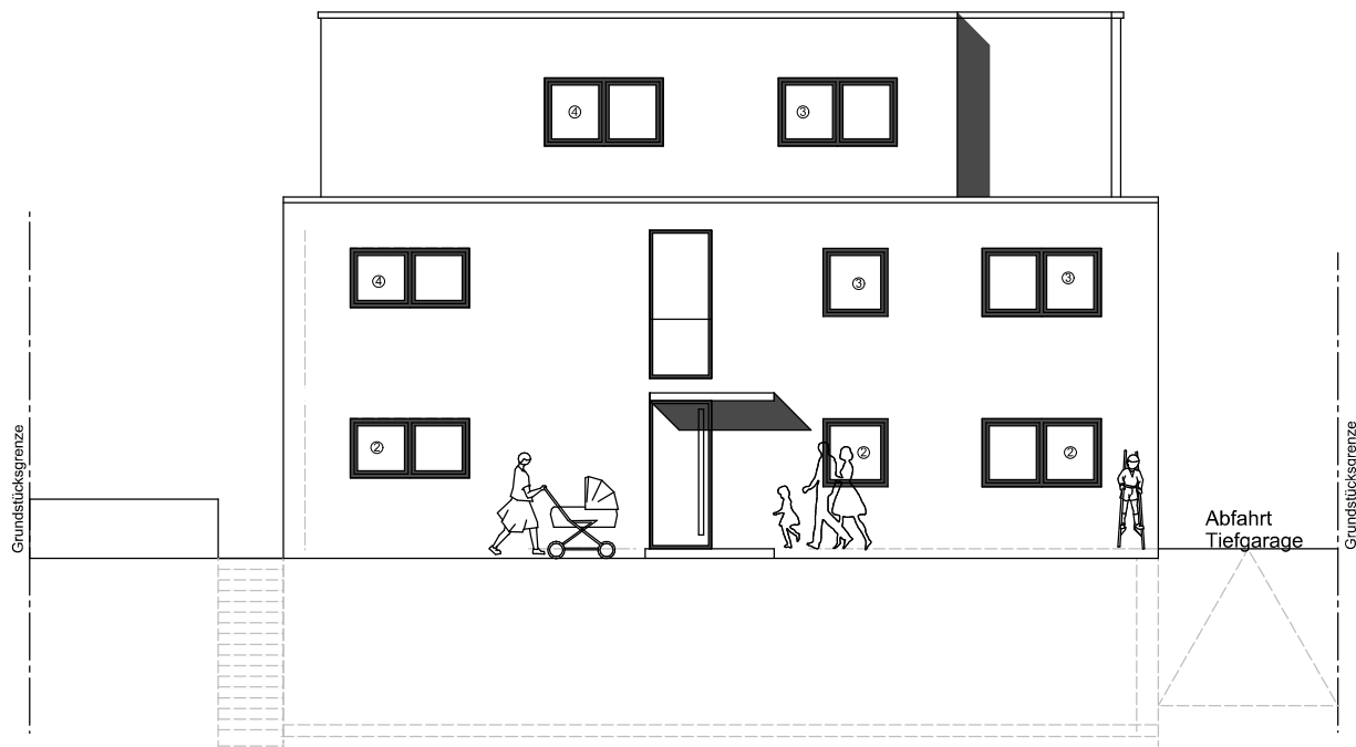
Ansicht Straße / Norden
